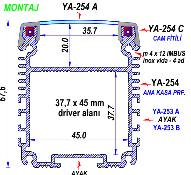
Wallwasher - Projektör Kasalarına uygun
