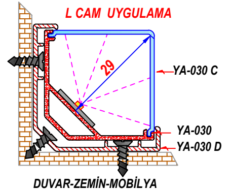
YA-030 C ye Uygun
