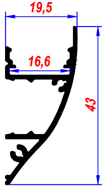
YA - 023 Alm.Led Kasa
