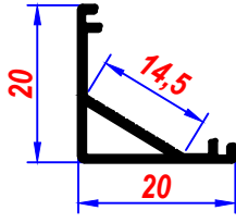
L KÖŞE Profili
