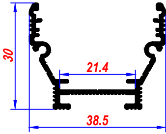
YA-201 C P.C. Difüzör Düşük Bombeli-Çizgili
