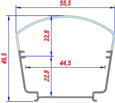
IP 66 KOEKS KÜÇÜK PC. KASA
