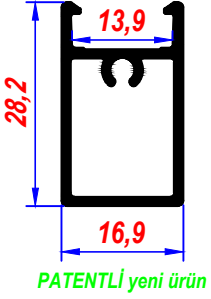
AVZ-015 Alm.Led-Avize Kasa
