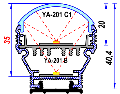
YA-202 D Duv.Bağlt. YA 201 C - YA 201 B1 Cam-Kızak uygulaması
