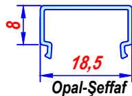
YA-001 A U P.C.Difüzör
