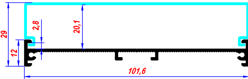
RK - 001 Alm. Reklam Yönlendirme / Led Pef.
