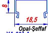
YA-001 A U P.C.Difüzör
