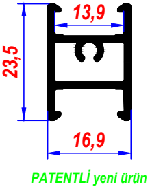
AVZ-017 Alm.Led-Avize Kasa
