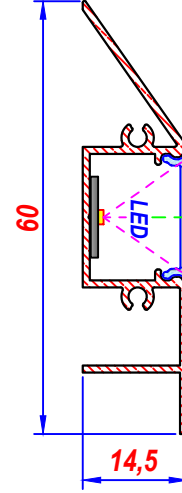
YA-093 Alm. Profil
