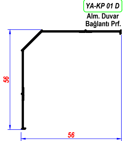
İSTENİLEN RENKDE ÜRETİLİR İSTENİLEN ÖLÇÜLERDE KESİM YAPILIR UYGULAMA
