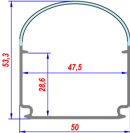
IP 66 KOEKS KÜÇÜK PC. KASA
