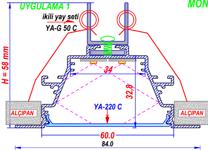
2 FARKLI TAVAN MONTAJ YAYI
