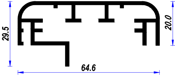
RK - 004 Alm. Kayan Yazı Reklamı Prf.
