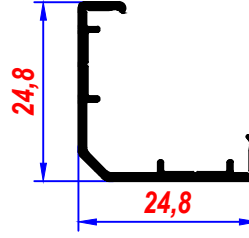
Alm. Duvar Bağlantı Prf.
