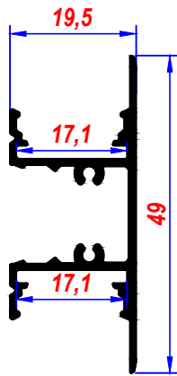
YA - 024 Alm.Led Kasa
